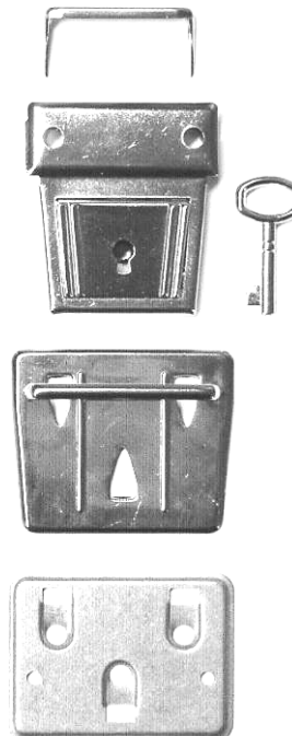
Art. Nr. 183 Metall, silber vernickelt, mit Schloß Steckerbreite: 31-36mm Beutel mit 10 Stück
